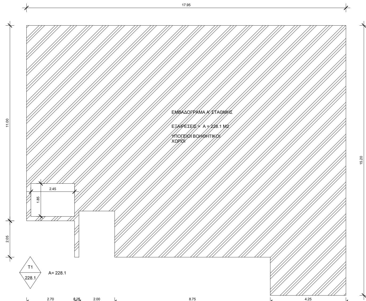
1 ΕΜΒΑΔΟΓΡΑΜΑ Α' ΣΤΑΘΜΗΣ 1 : 100
