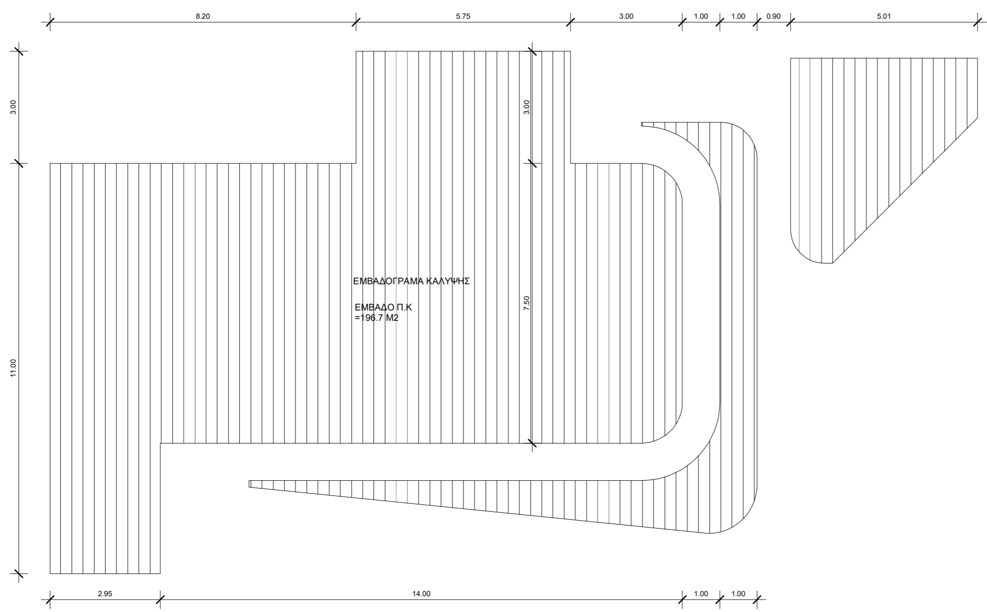
2 ΕΜΒΑΔΟΓΡΑΜΑ ΚΑΛΥΨΗΣ 1 : 100
