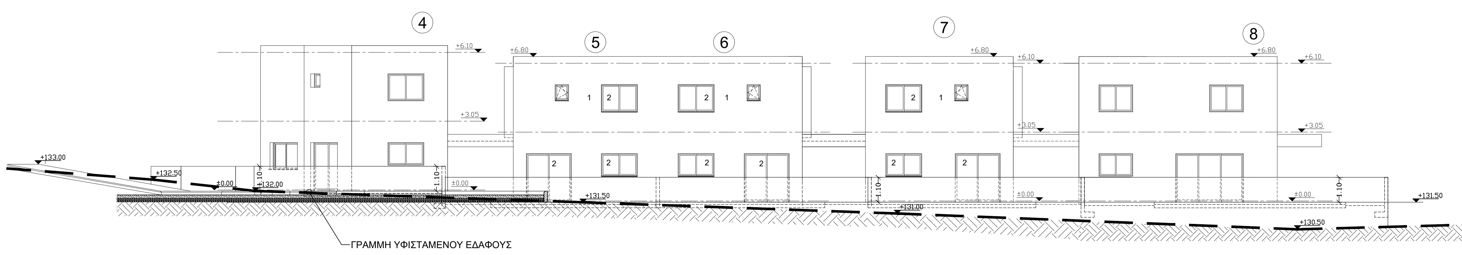
ΝΟΤΙΟΔΥΤΙΚΗ ΟΨΗ
