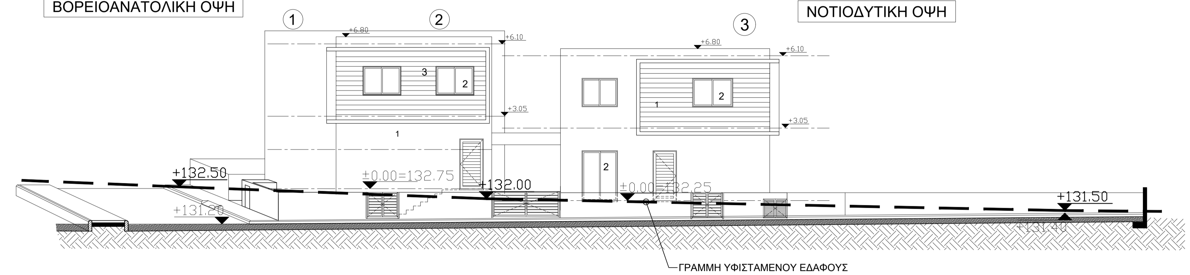
ΝΟΤΙΟΔΥΤΙΚΗ ΟΨΗ
