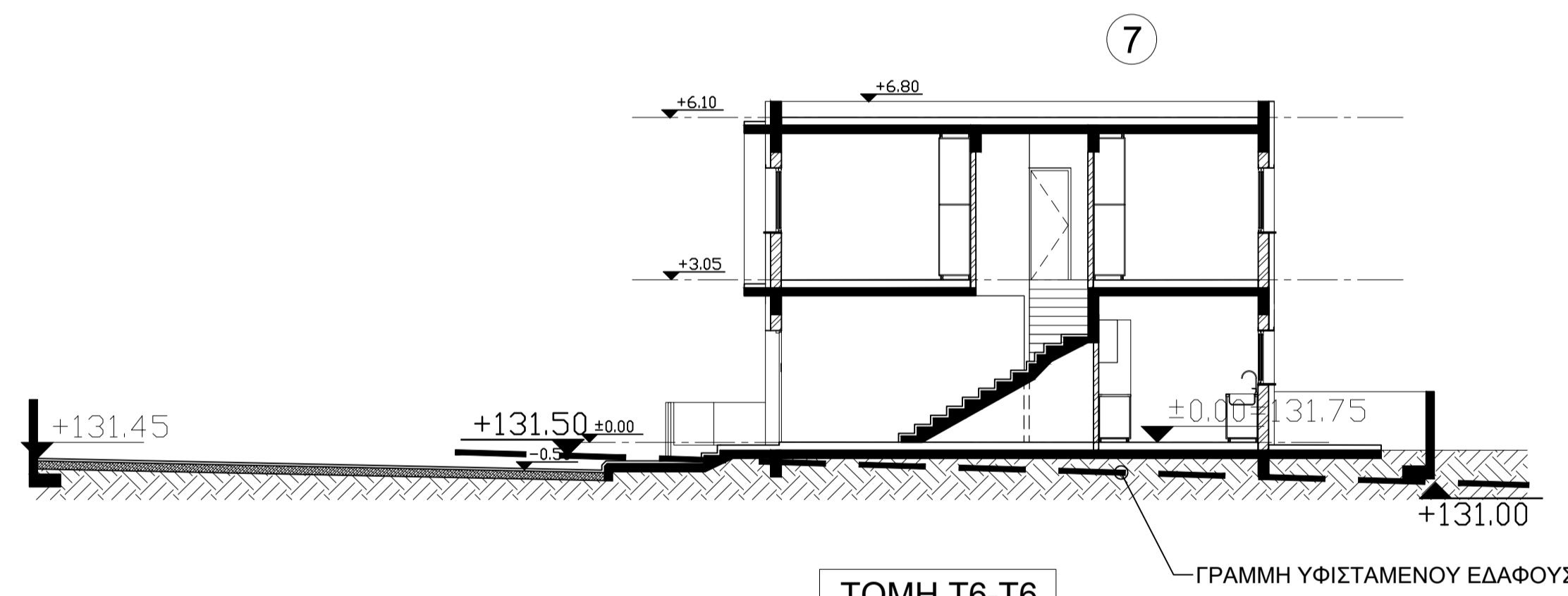
ΤΟΜΗ Τ6-Τ6
