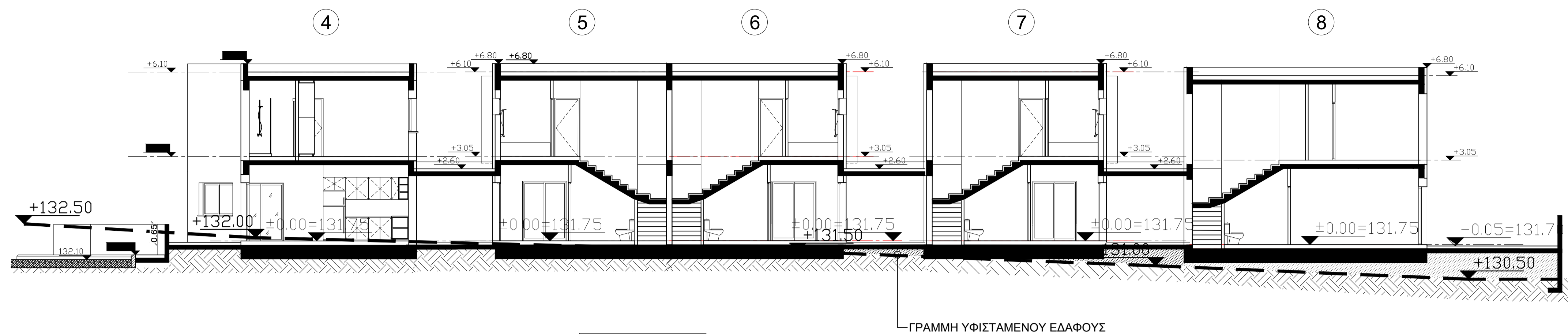
ΤΟΜΗ Τ1-Τ1
